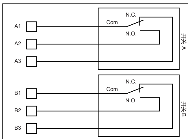
图31 辅助开关的端子图
